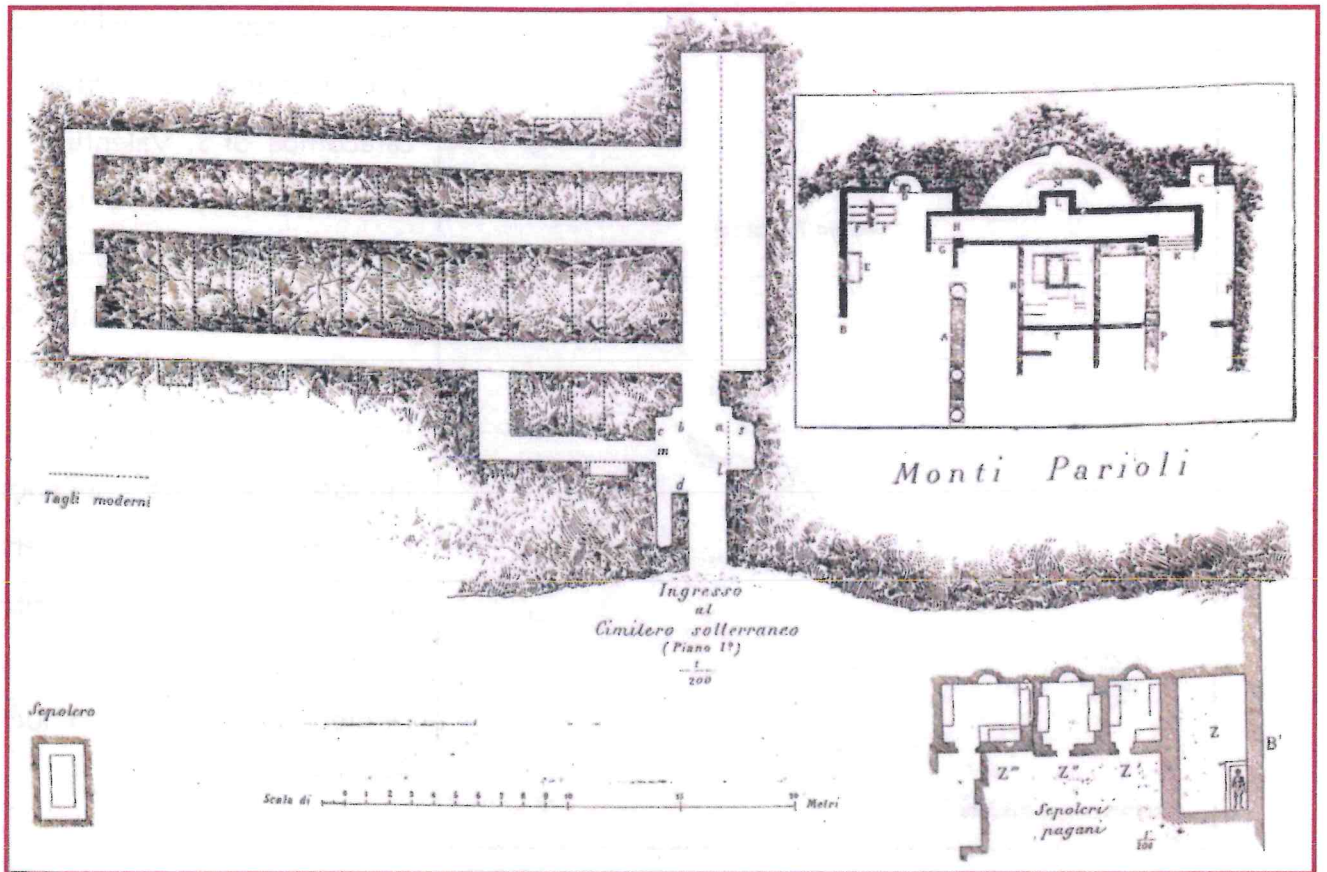
Fig. 7: Basilica e catacombe di S. Valentino (da MESSINEO 1991)
